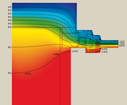
Disegno 3 - Serramento filo esterno muratura.
