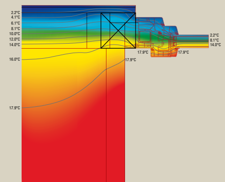
Disegno 4 - Serramento nel coibente.
