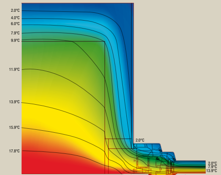
Disegno 1 - Serramento filo interno muratura.
