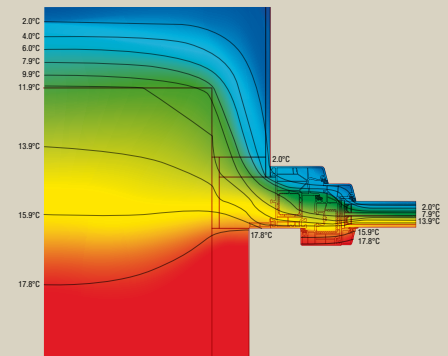
Disegno 2 - Serramento metà spalletta.
