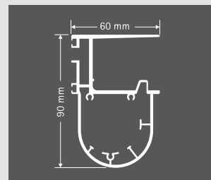
Guida orizzontale lato opposto al motore (standard è a sinistra, vista interna)
