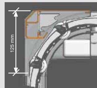
Guida orizzontale lato opposto al motore (standard è a sinistra, vista interna)
