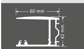
Guida verticale 60 per il montaggio in luce
