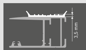
Profilo di tenuta per guida verticale 77
