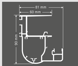
Guida orizzontale lato motore (standard è a destra, vista interna)
