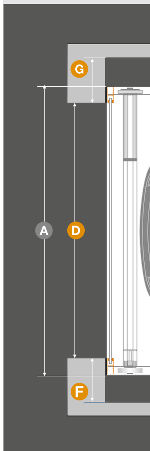
Guida divisa 110 x 44 mm
